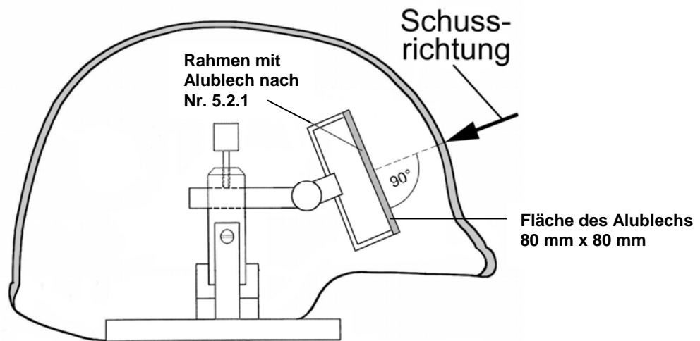
Seitenansicht
