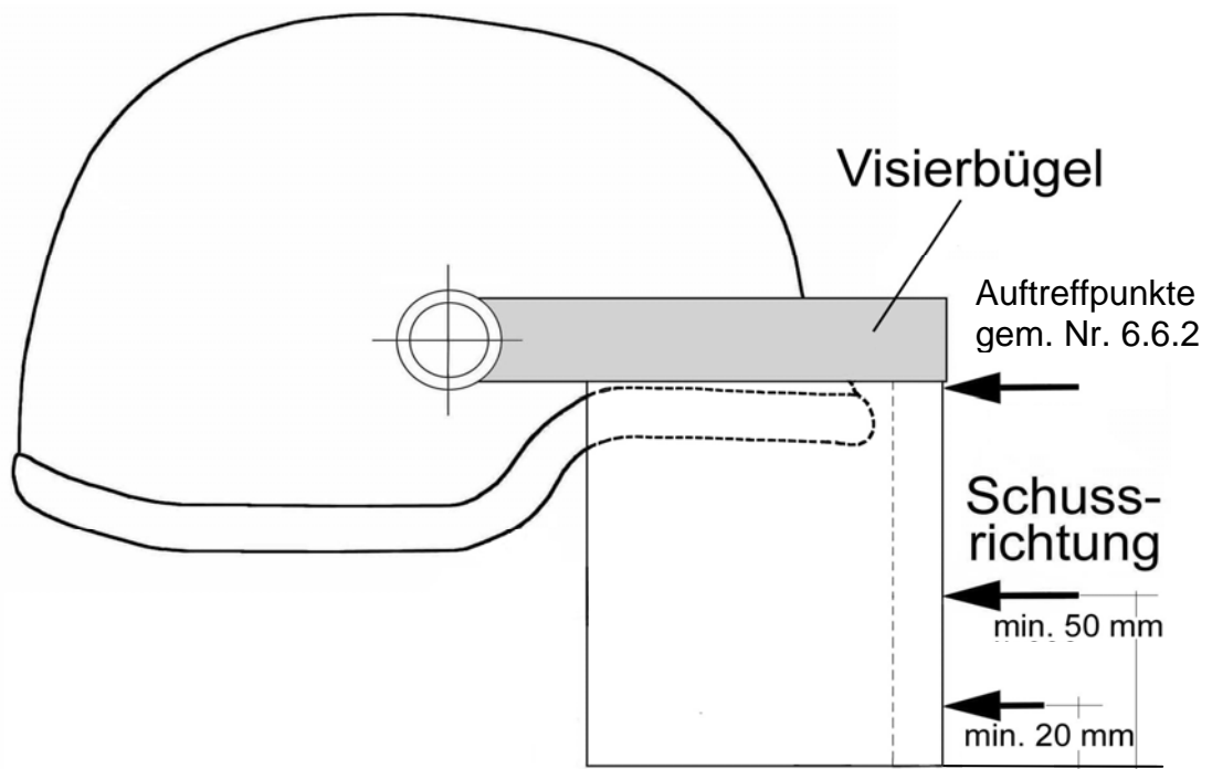
Seitenansicht
