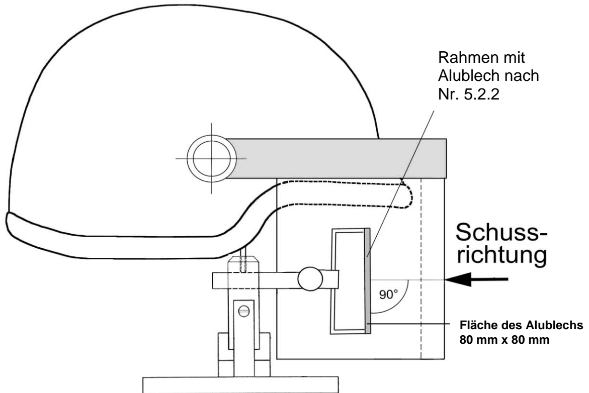
Seitenansicht schematisch
